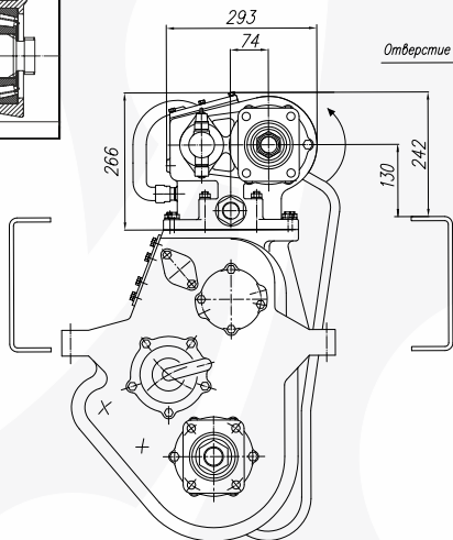
Раздаточные коробки 65111, 43114
